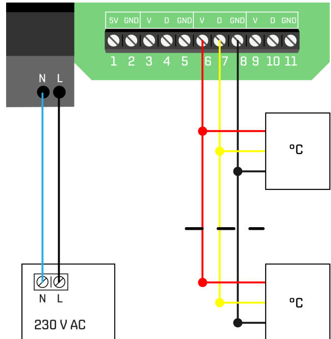
Rys. 1: Przykład podłączenia TCM Sensor T
